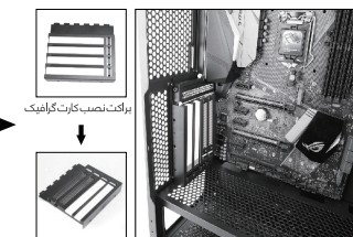
براکت کارت گرافیک را درون کیس نصب کنید
