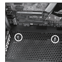
با استفاده از سر پیچ، پایه های مسی را در محل های علامت گذاری شده نصب کنید
