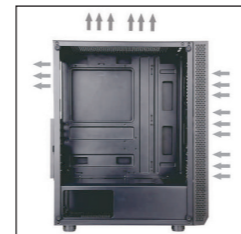
جهت صحیح ورودی و خروجی هوای کیس
