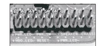
محل نصب نشانگر ها و کلید ها بر روی مادربرد
