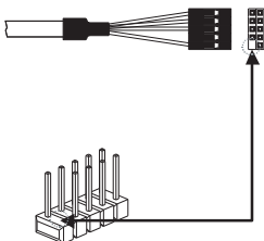
کانکتور USB 2.0 مادربرد
