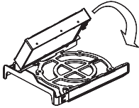
نحوه نصب هارد 3.5" (بدون نیاز به پیچ)
