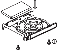
نحوه نصب هارد 2.5"
