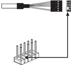
کانکتور صدای HD مادربرد
